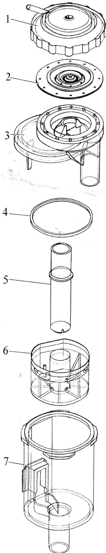
Рис.9 Приемник ПАД 03.000 СБ
