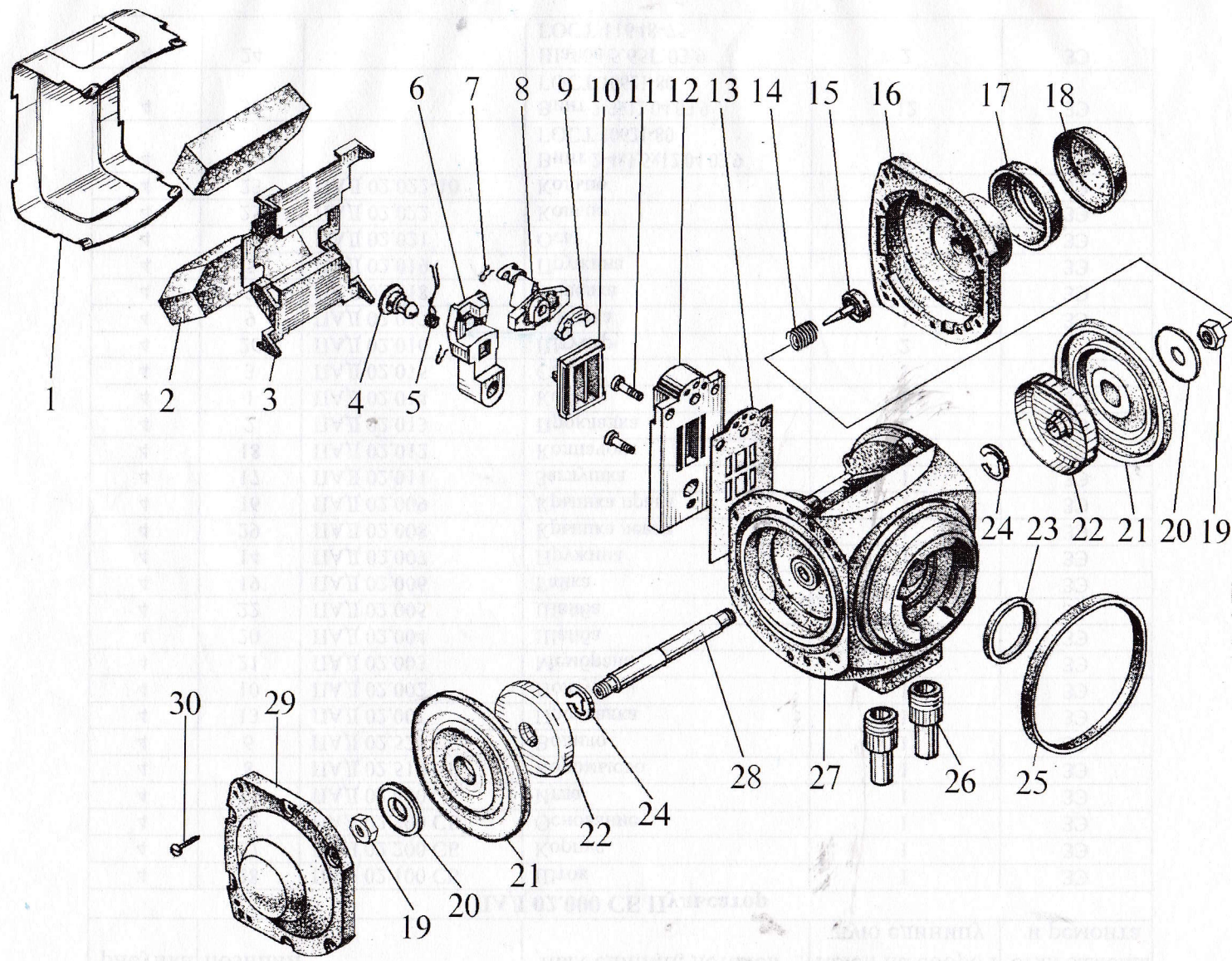
Рис.4. Пульсатор ПАД 02.000 СБ
